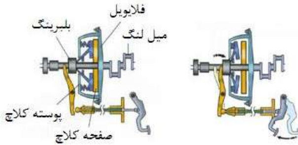
درگیری کلاچ با فلایویل (سمت چپ) و آزاد شدن کلاچ با فشردن پدال (سمت راست)
